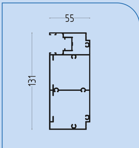
ΠΛΑΪΝΟ ΠΡΟΦΙΛ / SIDE COLUMNS - 5RAIL
