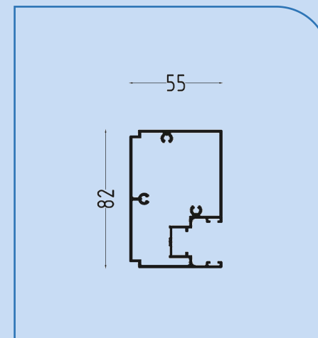
ΠΛΑΪΝΟ ΠΡΟΦΙΛ / SIDE COLUMNS - 3RAIL
