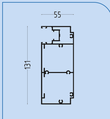
ΠΛΑΪΝΟ ΠΡΟΦΙΛ / SIDE COLUMNS - 4RAIL
